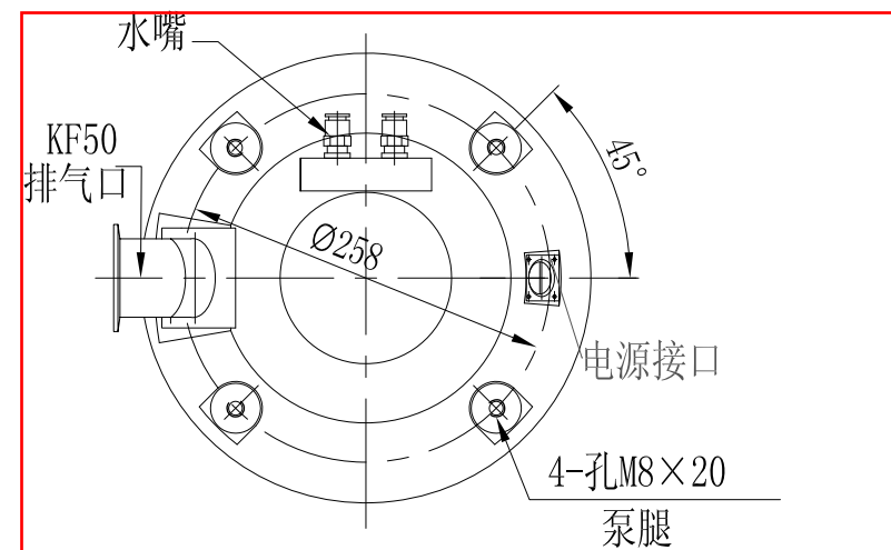
FF250/1600B分子泵安装尺寸图
